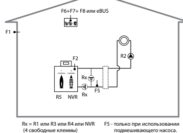
Схема №4 HZR-C
