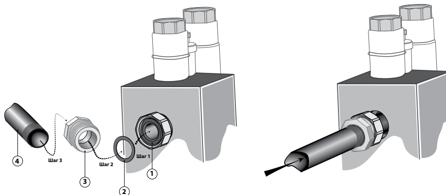
Элементы подключения трубопровода котлового контура к гидравлической стрелке «Поколение 8».
