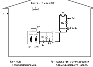
Схема №6 HZR-C
