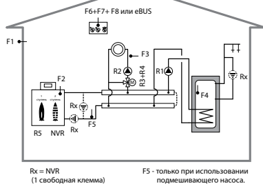
Схема №5 HZR-C
